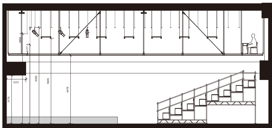
《劇場断面図》
