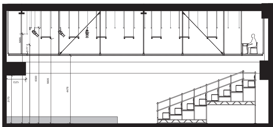
《劇場断面図》
